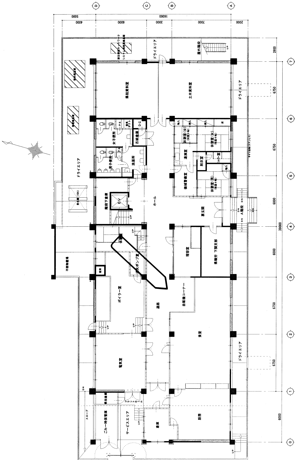
地階平面図
