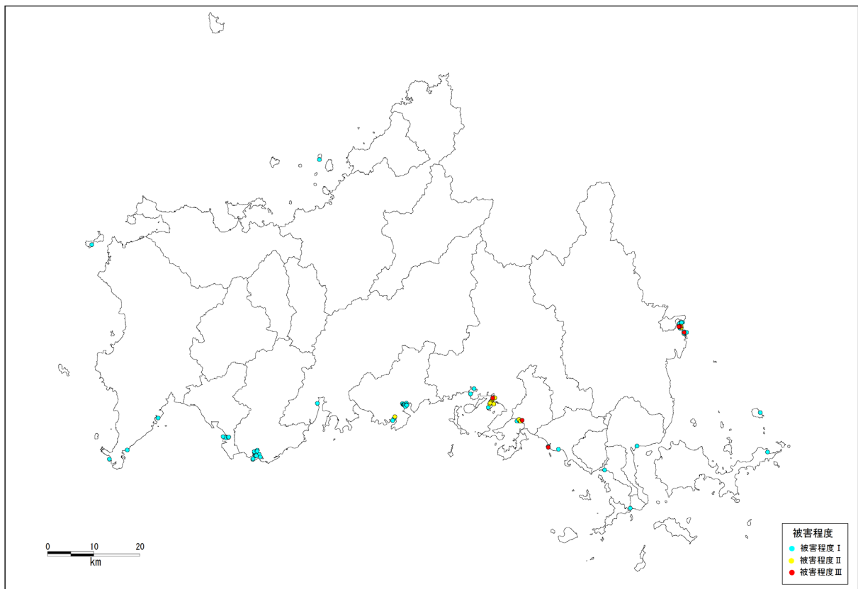
安芸灘～伊予灘の地震
