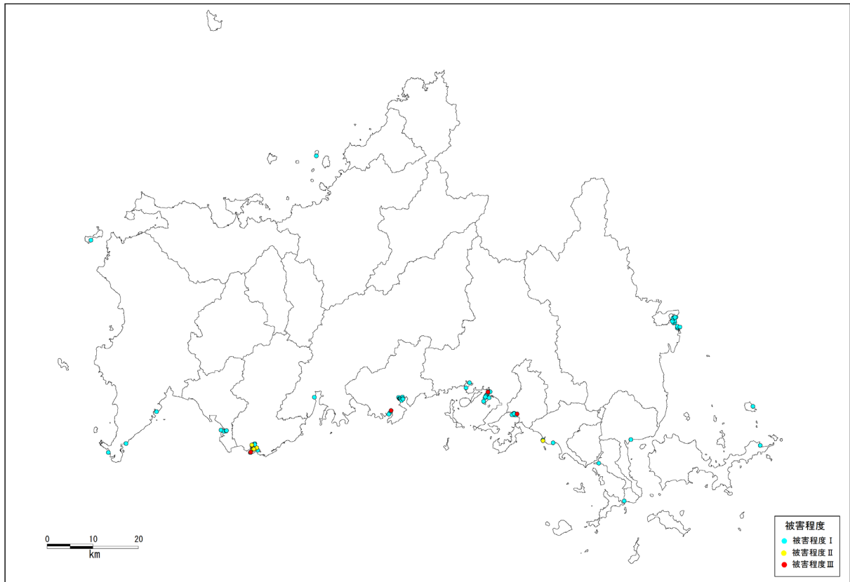
大原湖断層系（山口盆地北西縁断層）
