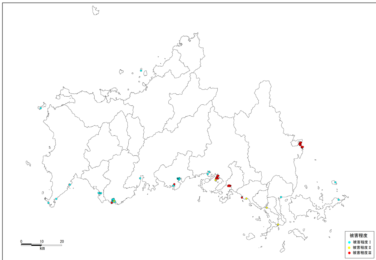
大竹断層（小方-小瀬断層）
