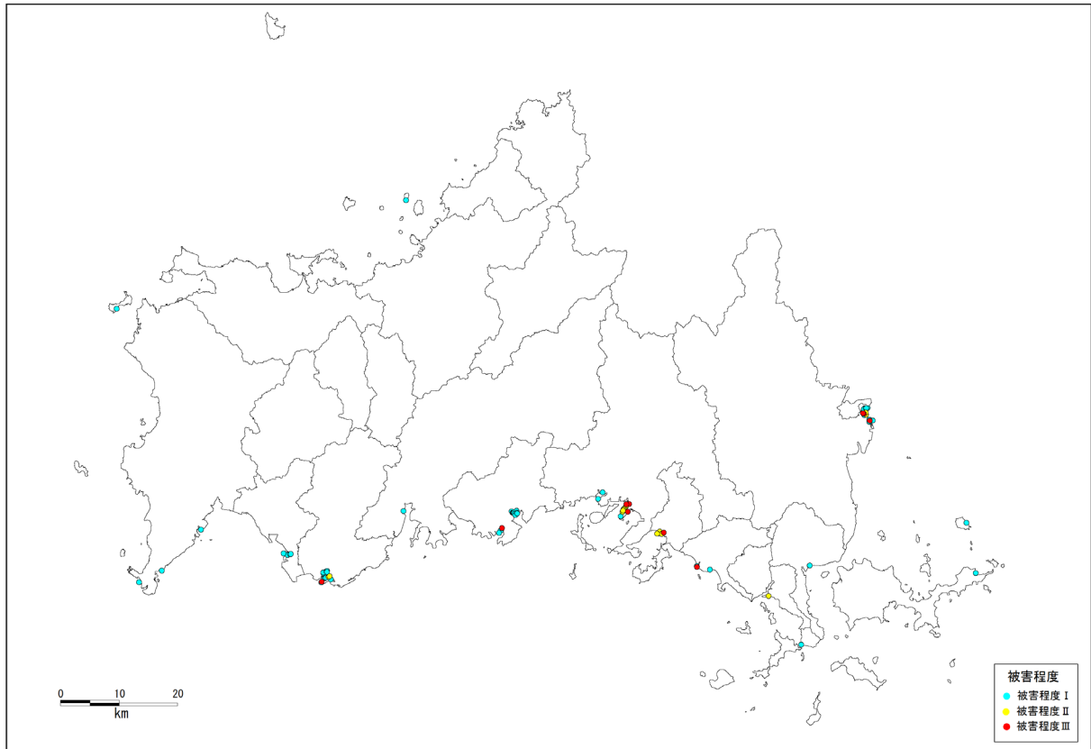
東南海・南海地震
