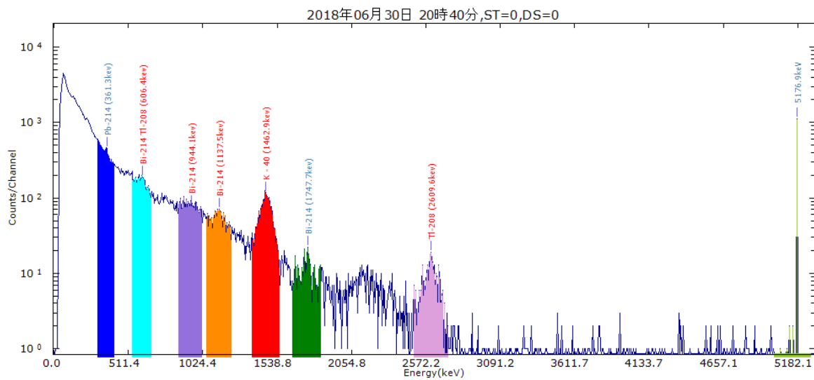
図2 平成30年6月30日 20:40 30.4nGy/h (最小値時のスペクトル)
