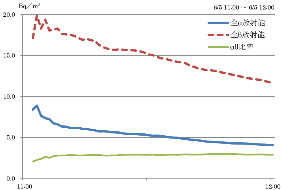
図3 全α・β放射能の減衰(6月5日)
