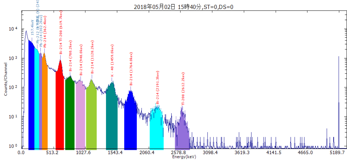
図1 平成30年5月2日 15:40 66.5nGy/h (最高値時のスペクトル)
