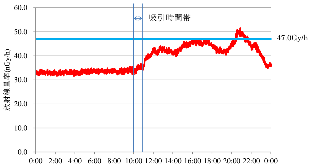
図4 空間放射線量率(6月5日)
