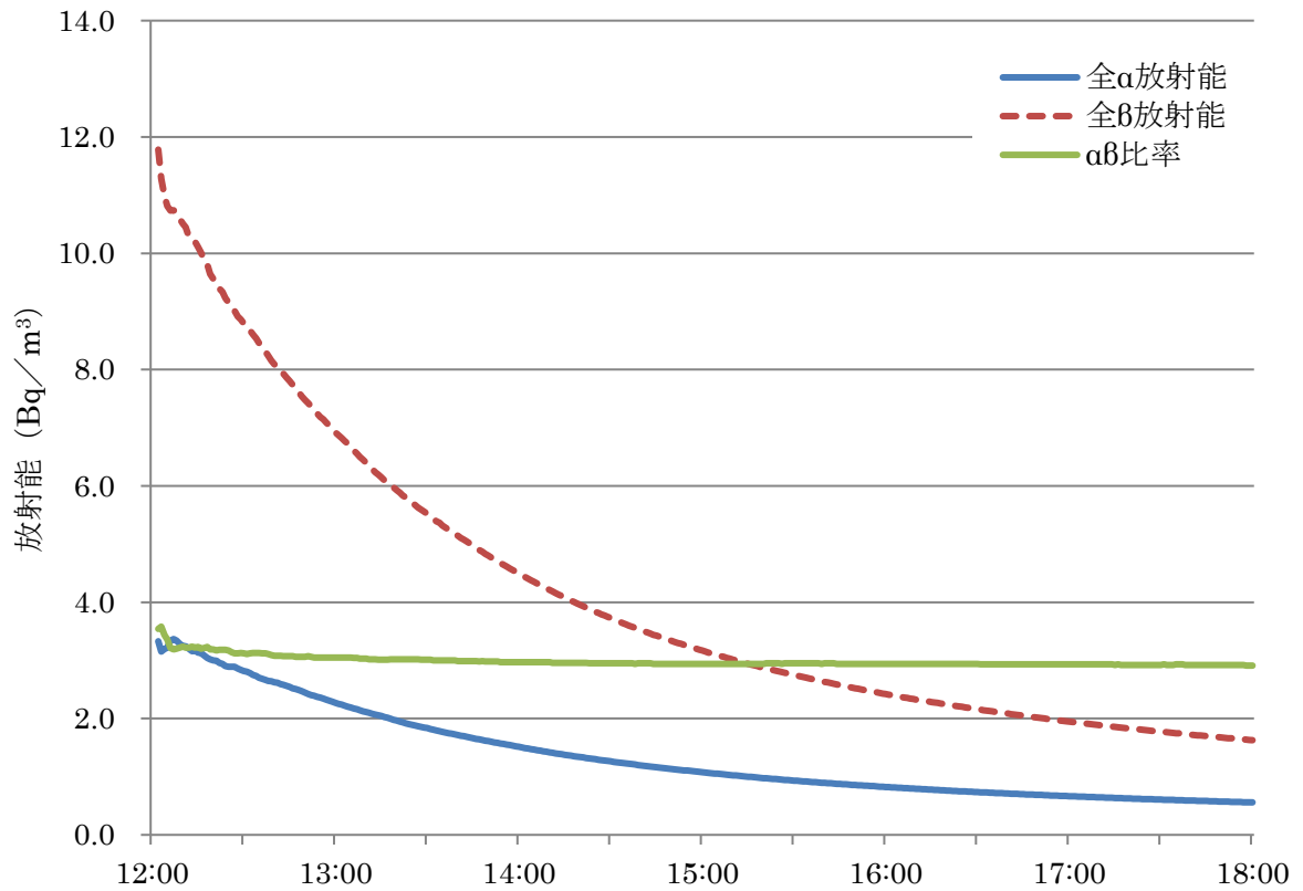
図4 全 \alpha ・ \beta 放射能の減衰(4月27日)
