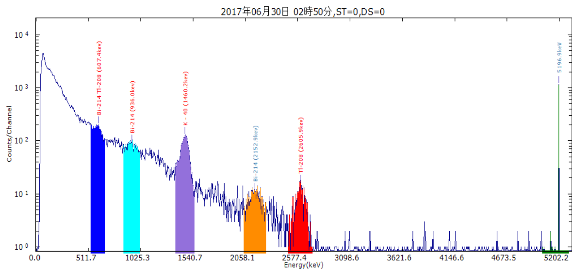
図2 平成29年6月30日 02:50 30.4nGy/h (最小値時のスペクトル)
