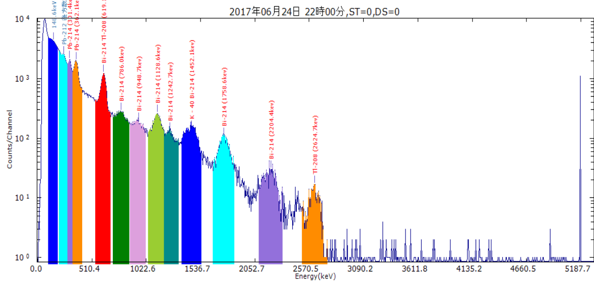
図1 平成29年6月24日 22:00 84.9nGy/h (最高値時のスペクトル)
