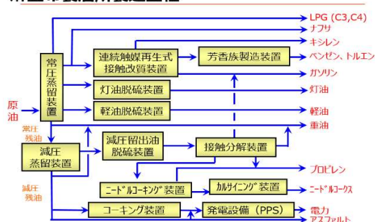
麻里布製油所製造工程
