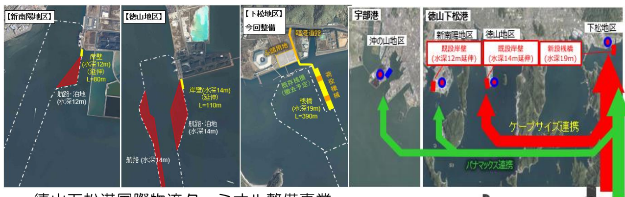
徳山下松港国際物流ターミナル整備事業
