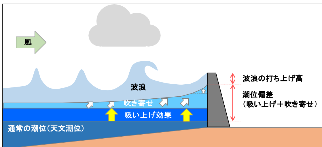
図 1.2 高潮発生メカニズム
