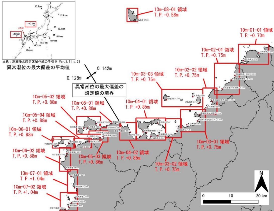
図 3.10 潮位の設定
