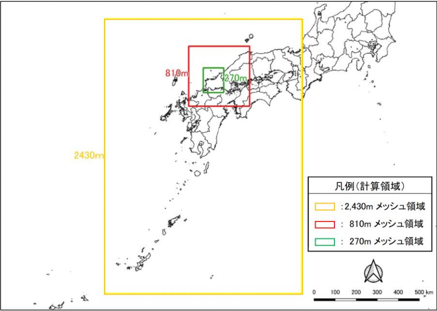
図 5.1 計算領域及び計算格子（広域）
