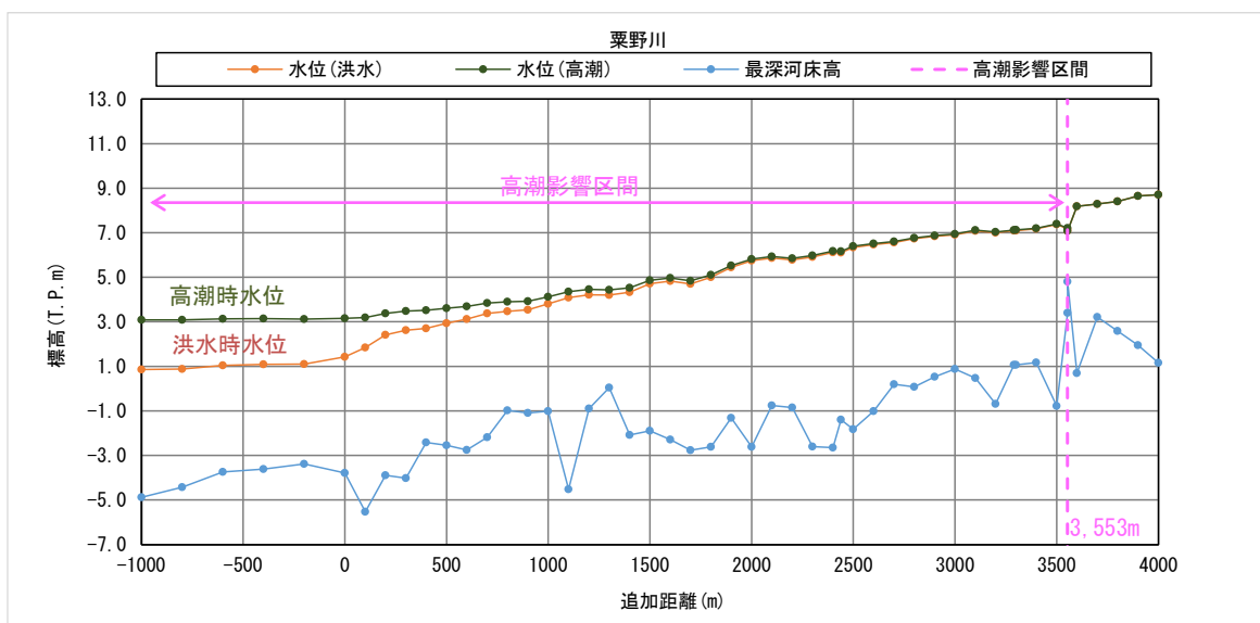
図 3.7 高潮影響区間の算定結果（粟野川の例）
