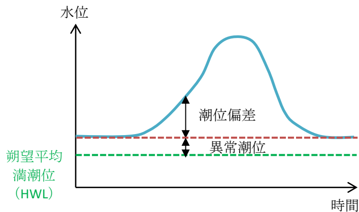
図 3.11 設定潮位の概念
