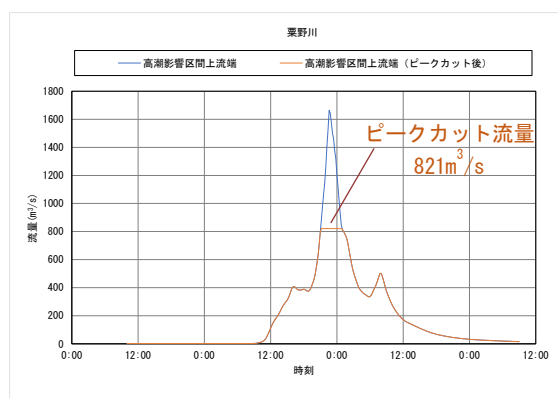
図 3.8 流量ハイドログラフ
