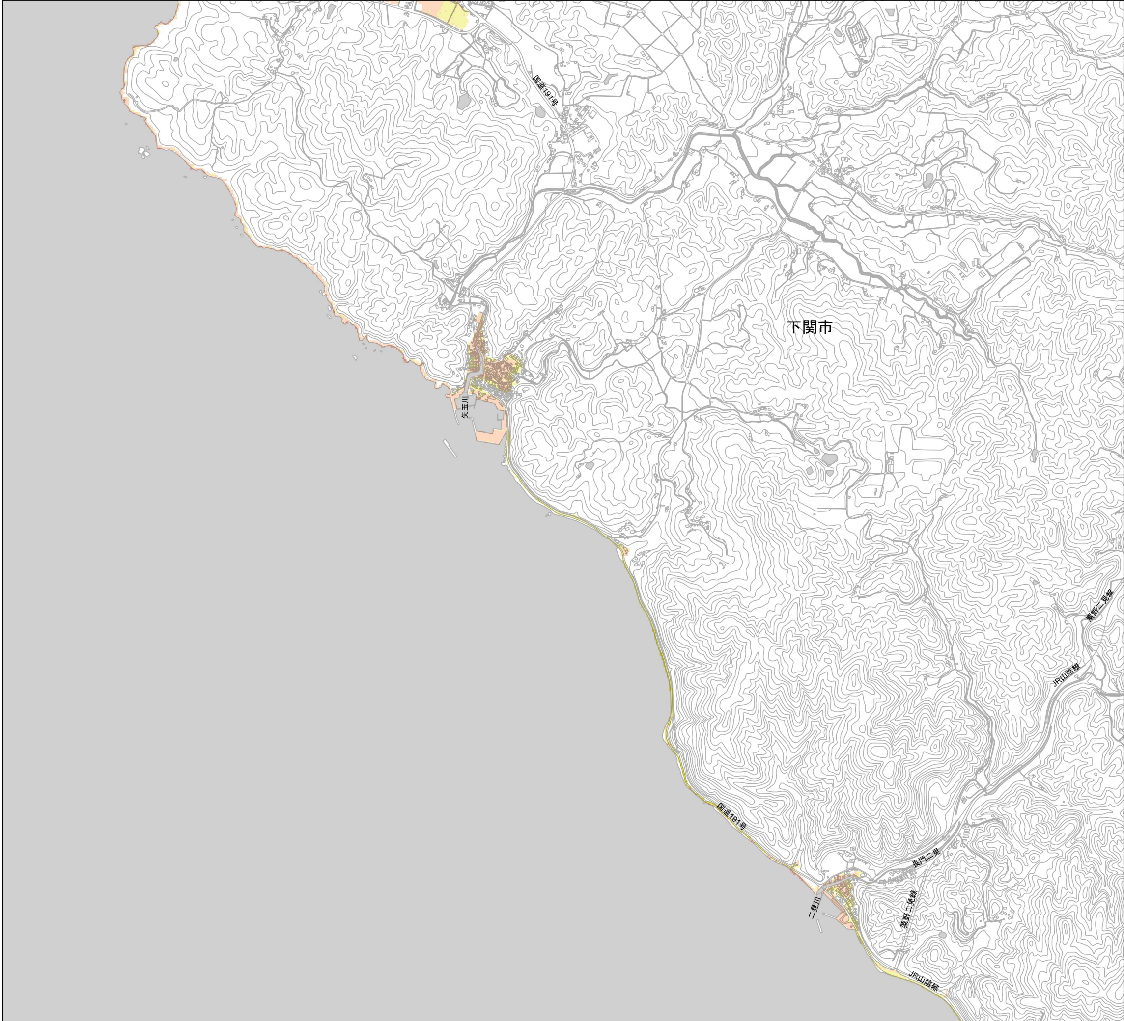
山口北沿岸 高潮浸水想定区域図 31（浸水深）
