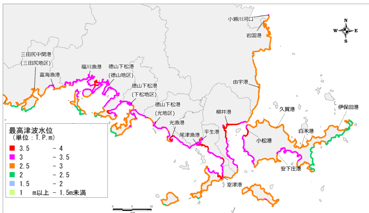
図4 最高津波水位分布（東部）
