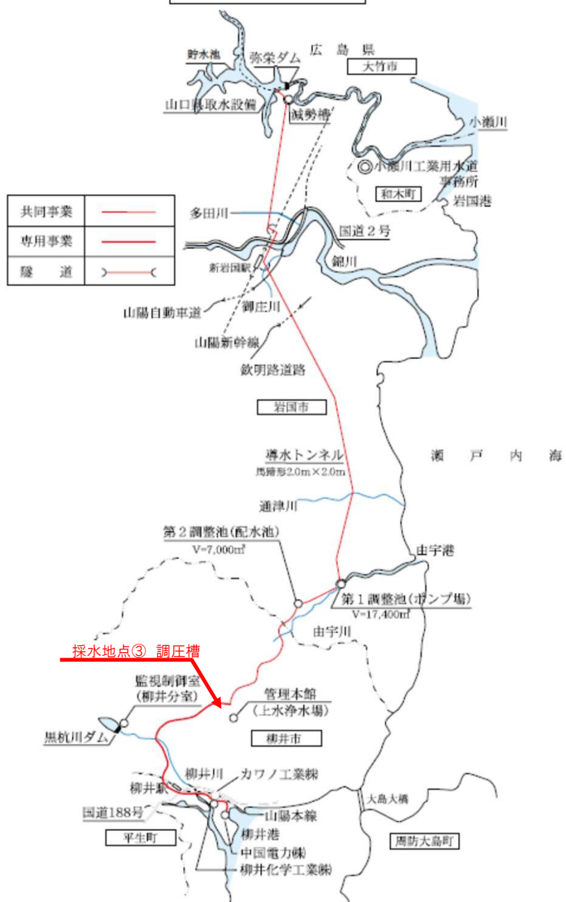
小瀬川第2期工業用水道概要図
