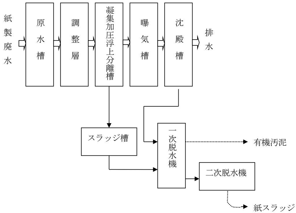
図1 排水処理フロー図
