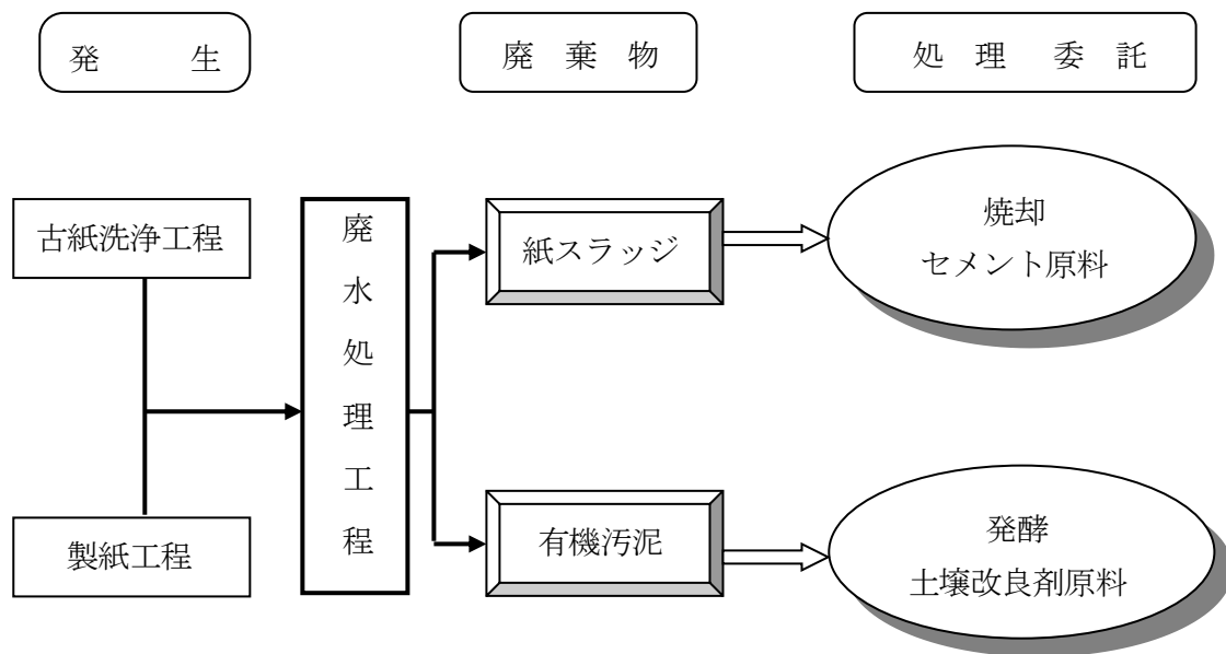
図2 廃棄物処理フロー図
