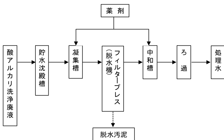
酸アルカリ排水処理施設〔No. 3〕
