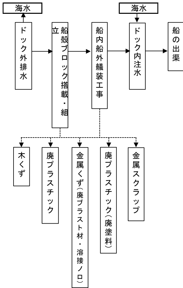
新造船建造フローシート [No. 1]
