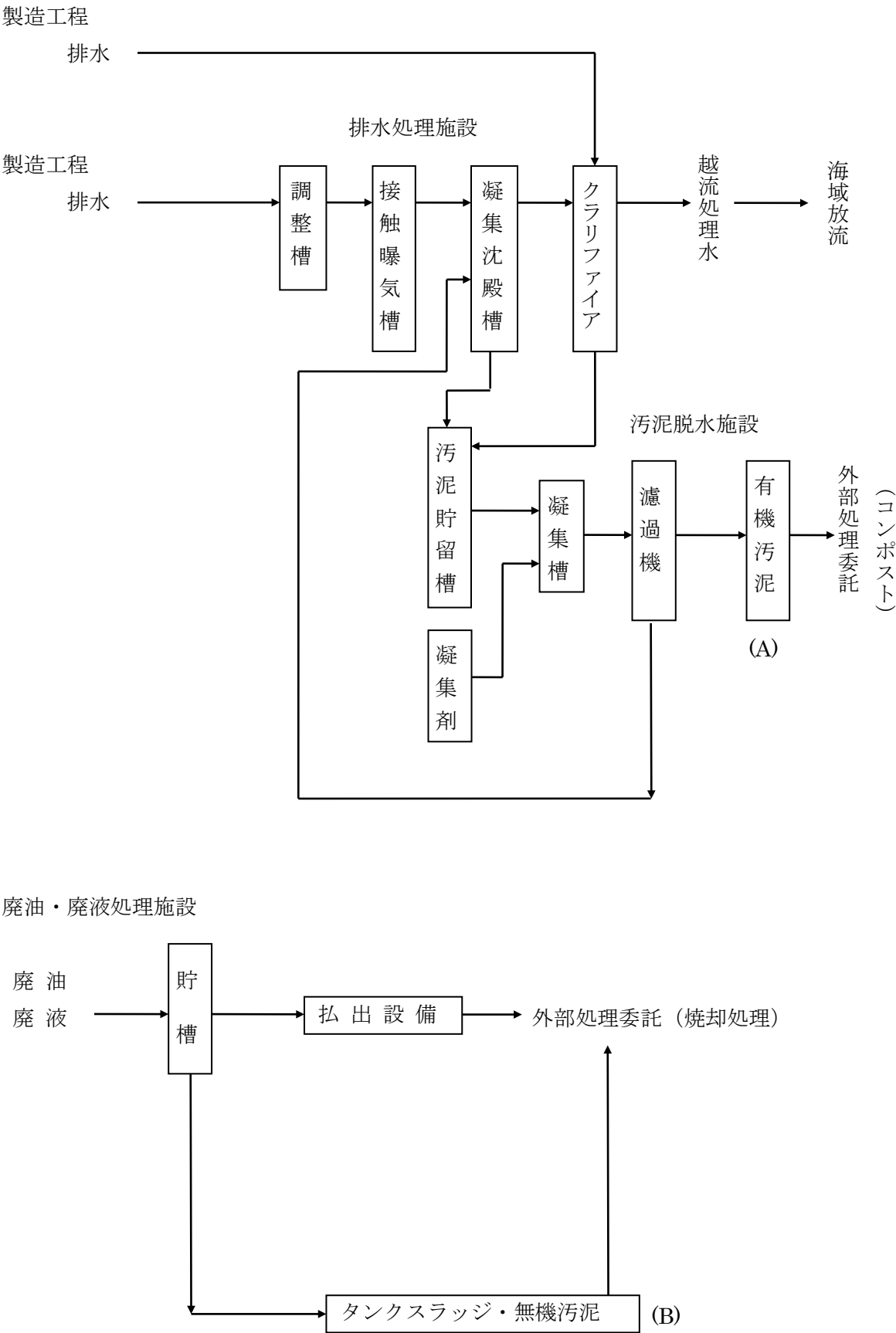
図4 廃棄物処理工程フローシート (No.4-1)
