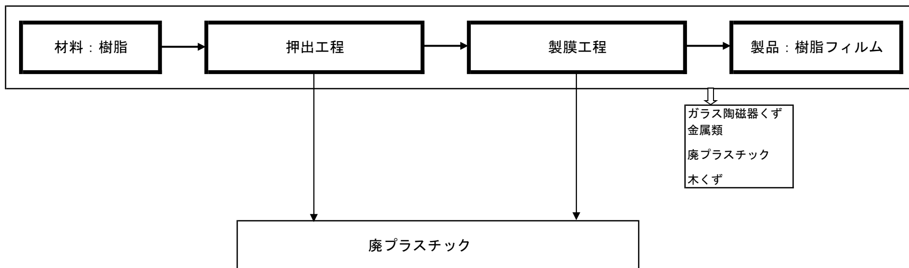
樹脂フィルム製造フローシート
