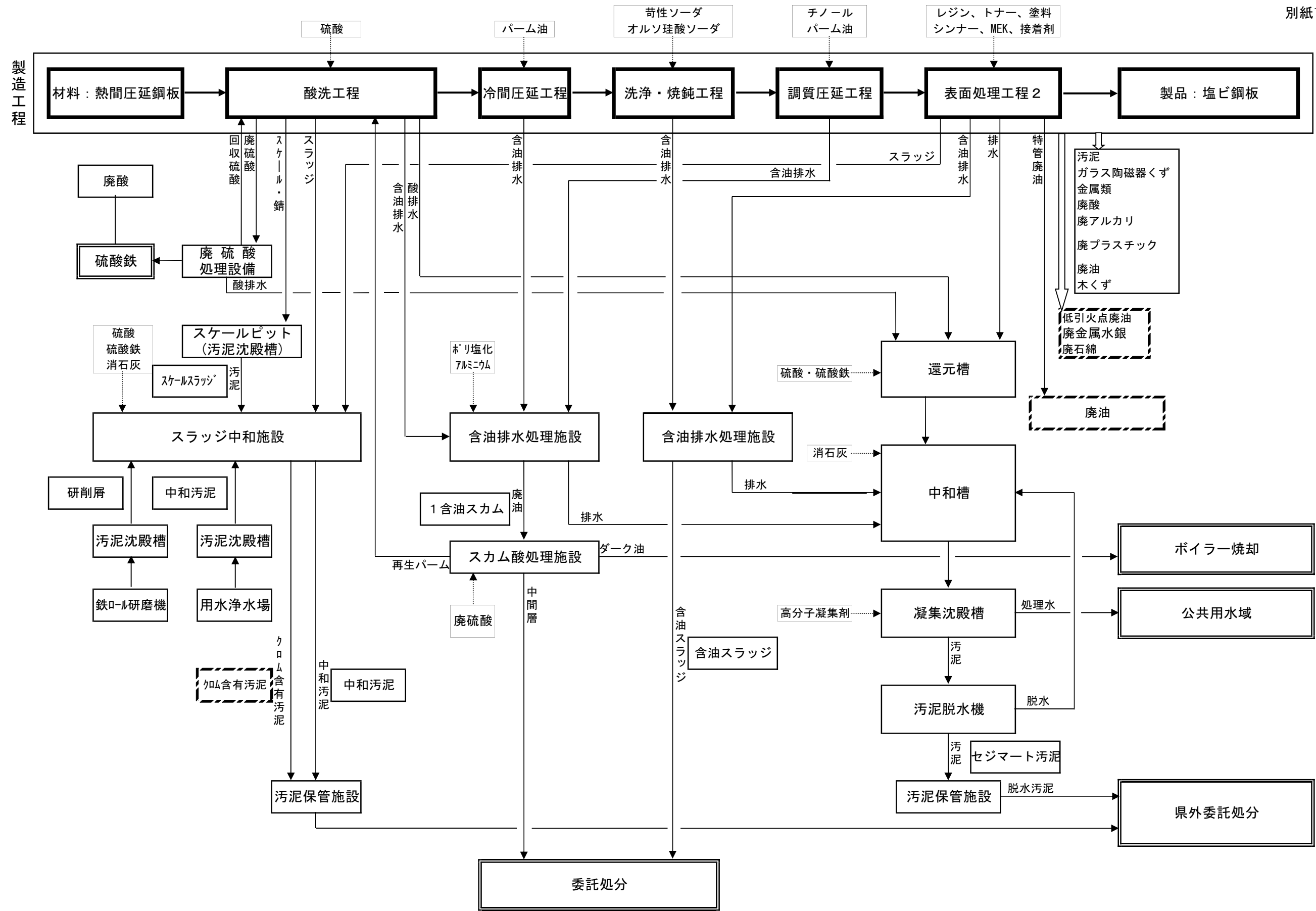
塩ビ鋼板製造フローシート ( 特別管理産業廃棄物 )
