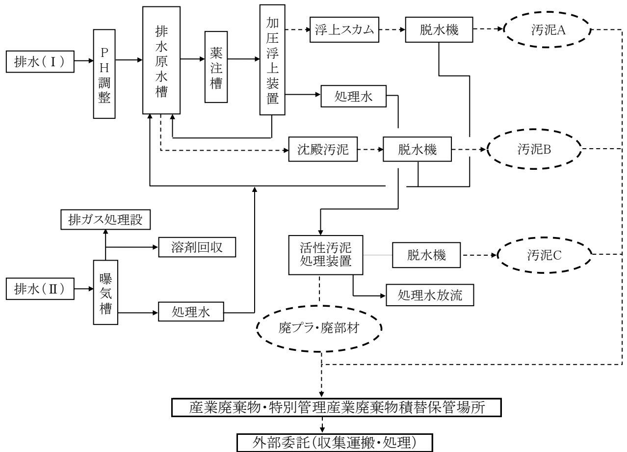
図5 排水処理工程に係る産業廃棄物発生・処理フロー(No. 5)
