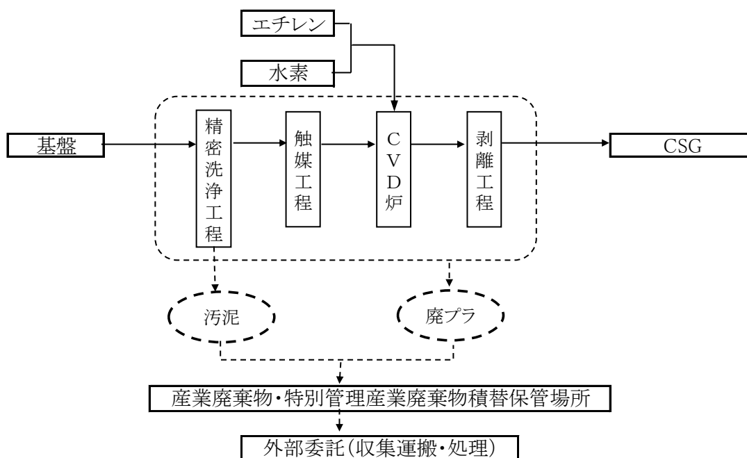
図4 CSG製造に係る産業廃棄物発生・処理フロー(No. 4)
