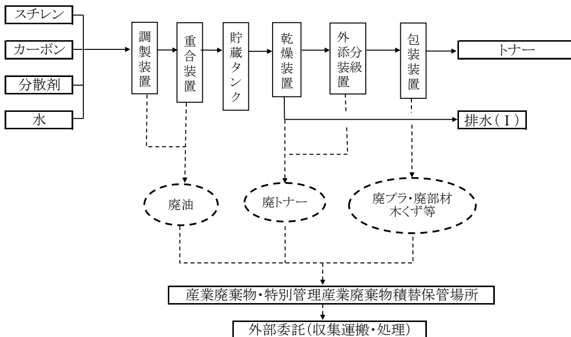
図3 トナー製造に係る産業廃棄物発生・処理フロー(No. 3)
