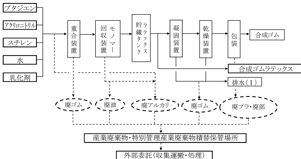
図1 乳化重合ゴム・合成ゴムラテックス製造に係る産業廃棄物発生・処理フロー (No. 1)
