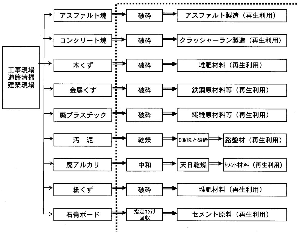
図1 廃棄物処理フロー図（現状）
