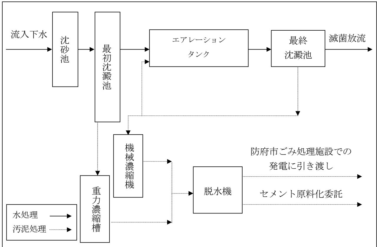
図1 産業廃棄物処理工程図
