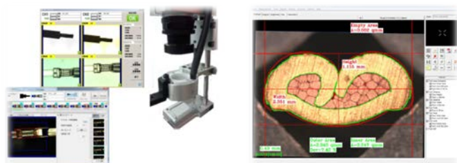
画像検査装置付の最新自動化システム クリンプ断面画像分析システム
