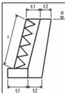
【法長、厚み等】
