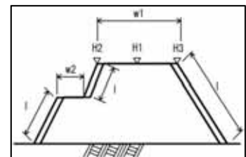
【法長等】
