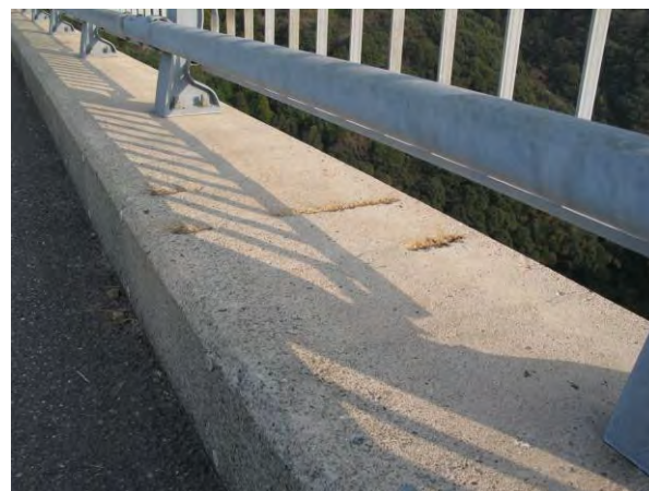
【かぶり不足のコンクリート構造物で発生した鋼材腐食の例】
