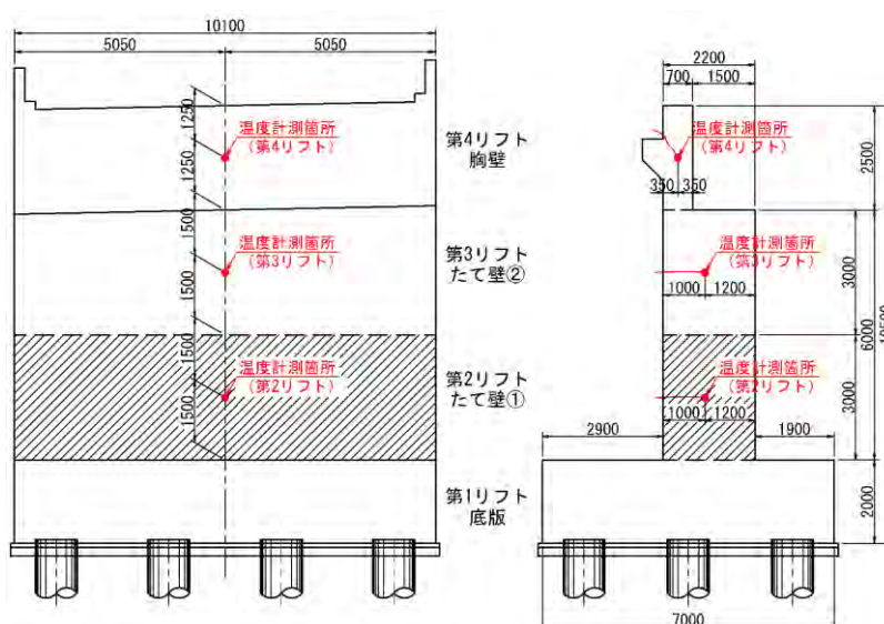
正面図
