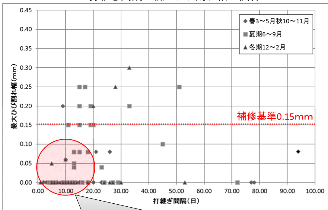
打継ぎ間隔と最大ひび割れ幅の関係
