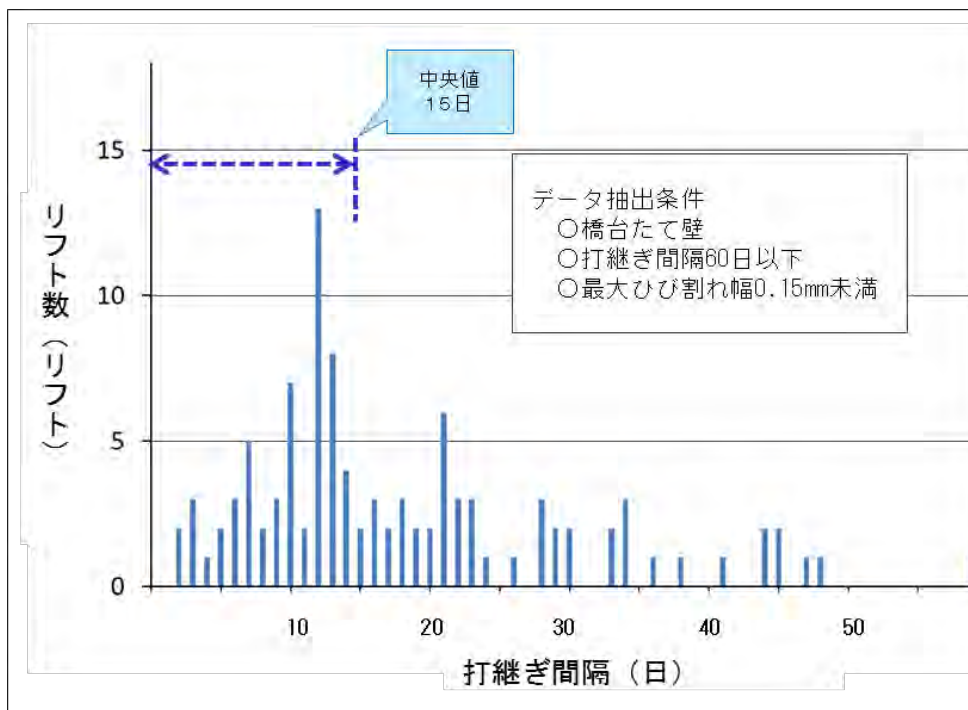
図 3.3.10 打継ぎ間隔と最大ひび割れ幅が0.15mm未滿のリフト数
