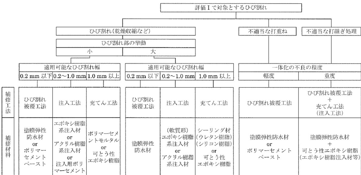
図 4.6.1 ひび割れの補修工法の選定例
