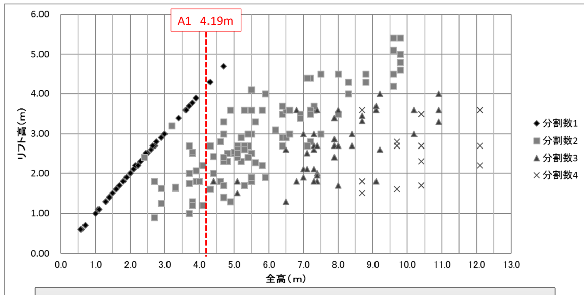
たて壁全高とリフト高(分割数)の関係
