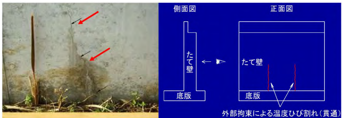
図 4.5.1 貫通ひび割れ
