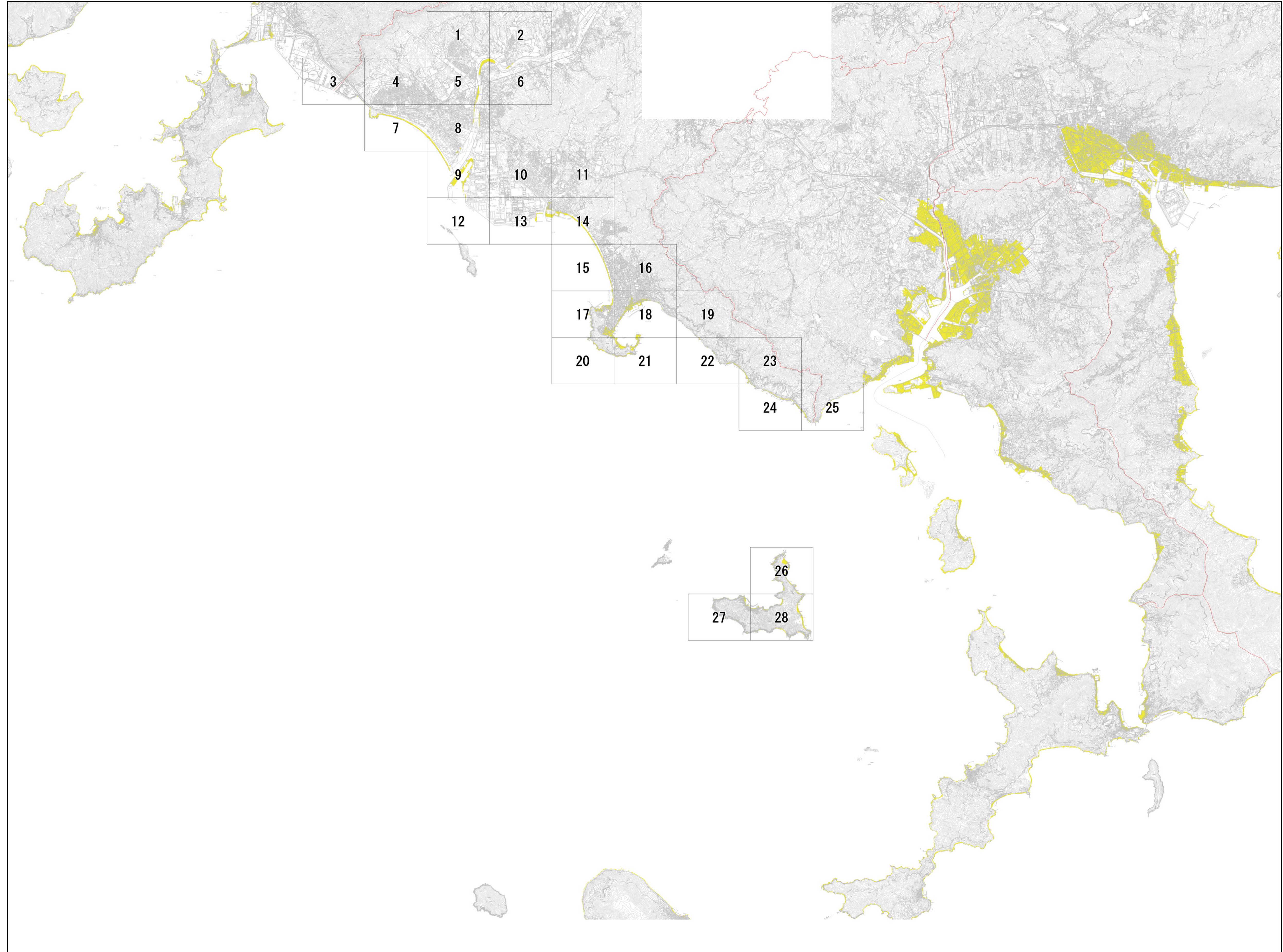
光市津波災害警戒区域位置図 A1版 1:50,000
