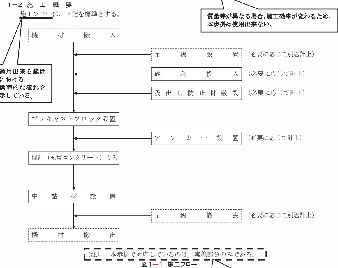
図1-1 施工フロー
